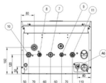
VISTA INFERIORE
